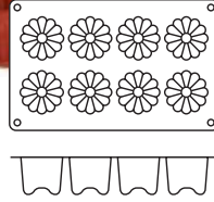
14.10058 SF050 8 big bordelais, 92 ml (5,5 cm | 5 cm) 17,3x29,7 cm pack: 1
